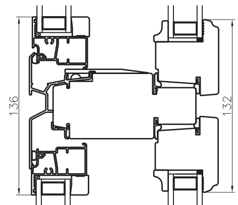
Vaakajakokarmi
