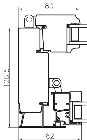
Sivukarmi
