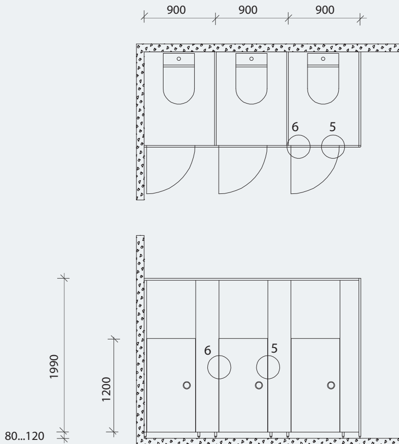
LASTEN WC 1:50
