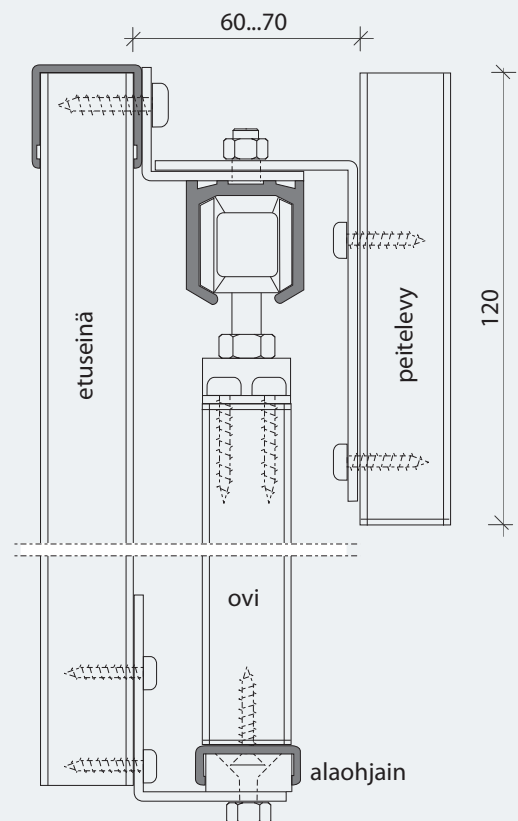
LIUKUOVI 1:2
