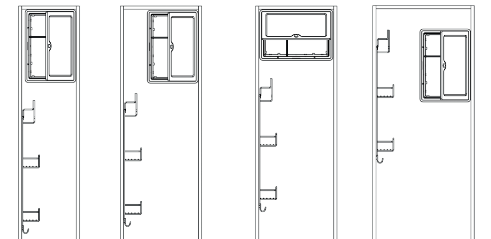
Lukittavan kaapin asennus pystyyn tai vaakaan (kuvan 400 mm leveässä komerossa myös vaakaan asennettuna)
