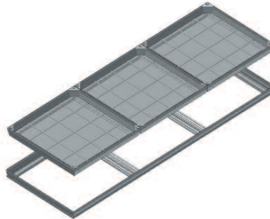
Sarjakansisto Kaksi tai useampia vakiokansia peräkkäin. Kansien välissä irrotettava tiivistyskisko.
