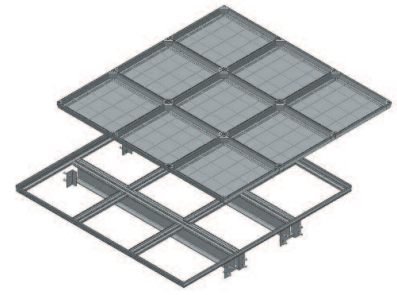
Yhdistelmäkansisto Yhteisessä kehyksessä kaksi tai useampia sarjakansistoja rinnakkain ja niiden välissä irrotettava kannatinpalkki sekä kansien välissä irrotettavat tiivistyskiskot.
