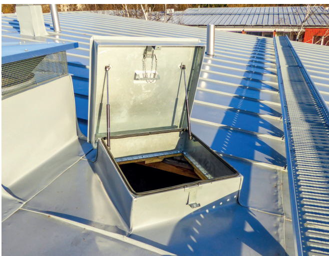
Kattoluukku konesaumakatoille
