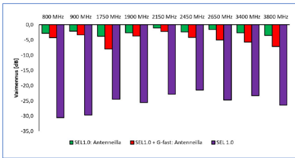
Kuva 4. Antennilasin vaimennus langattomille signaaleille mitattiin sekä yhden selektiivilasin (SEL1.0), että kahden selektiivilasin läpi (SEL 1.0 + G-fast).
