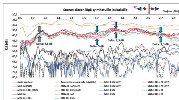
Kuva 2. Laboratoriomittauksissa havaitaan, että antennilasi-rakenne toimii lähes samalla tasolla riippumatta selektiivilasien määrästä. Yleensä selektiivilaseja on ikkunoissa 1-3 kpl.
