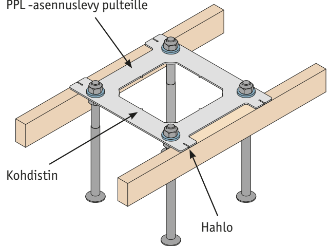
PPL –asennuslevy pulteille
