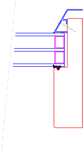
Leikkaus A -A, C-C
