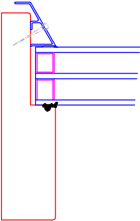
Leikkaus B -B
