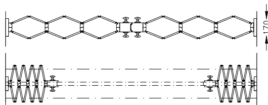
2-osainen taiteovi
