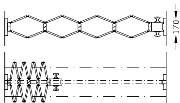
1-osainen taiteovi
