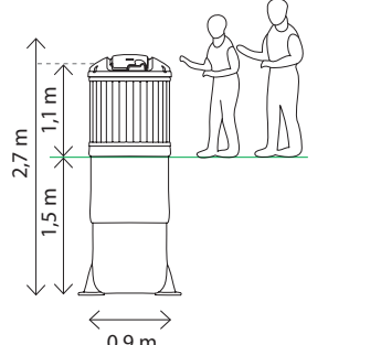
Molok®Classic 1,3 m³
