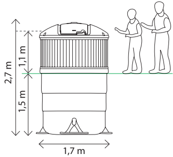
Molok®Classic 5 m³
