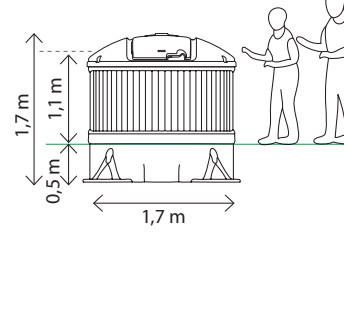
Molok®Classic Plus
