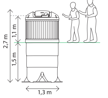
Molok®Classic 3 m³
