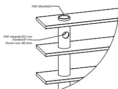
PSP VETOPUTKI
