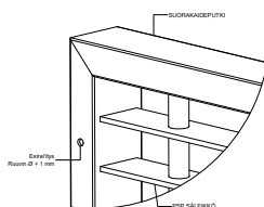
PUTKIKEHYS ETUKIINNITYS
