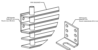
PSP KIINNIKE
