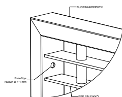
PUTKIKEHYS SIVUKIINNITYS
