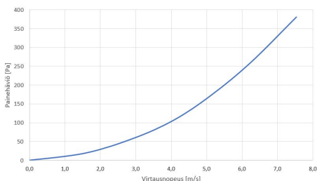
US-3B säleikkö C-50 (850mmx850mm)
