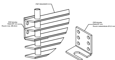
PSP KIINNIKE
