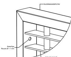
PUTKIKEHYS SIVUKIINNITYS
