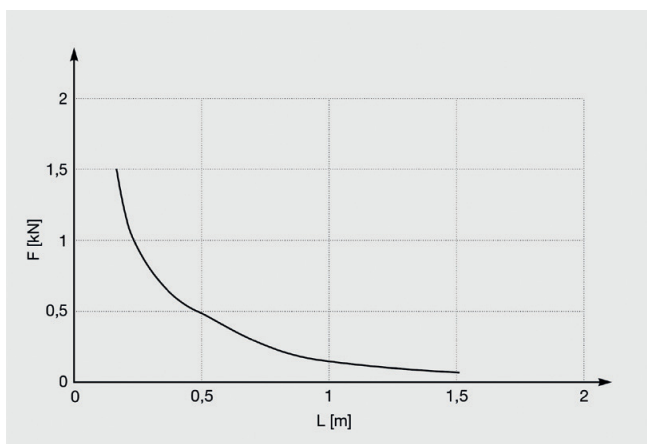
Asennuskisko 27/15
