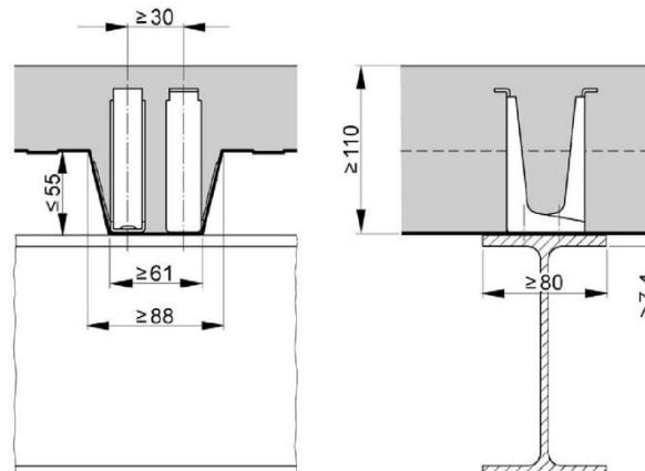
2 X-HVB alternés et centrés dans la nervure
