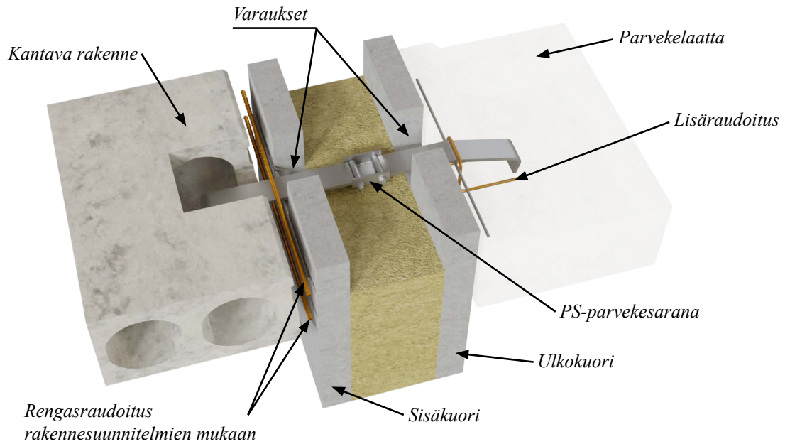
Kuva 2. PS-parvekesarana liitoksessa.
