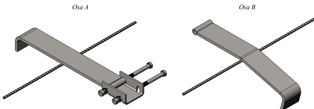
Kuva 4. PS-parvekesaranan osat.
