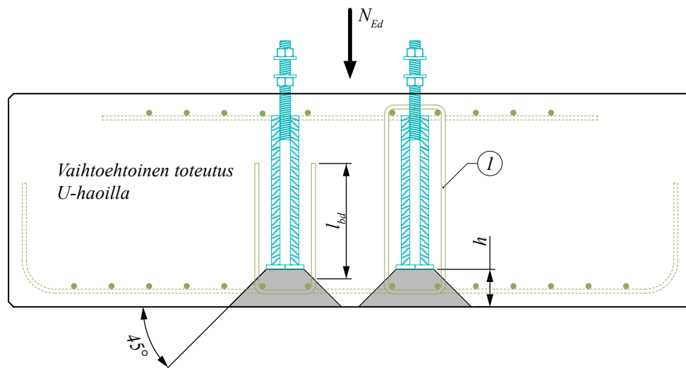
Kuva 12. Pultin tyssäkannan alle muodostuvan lävistyskartion raudoittaminen.
