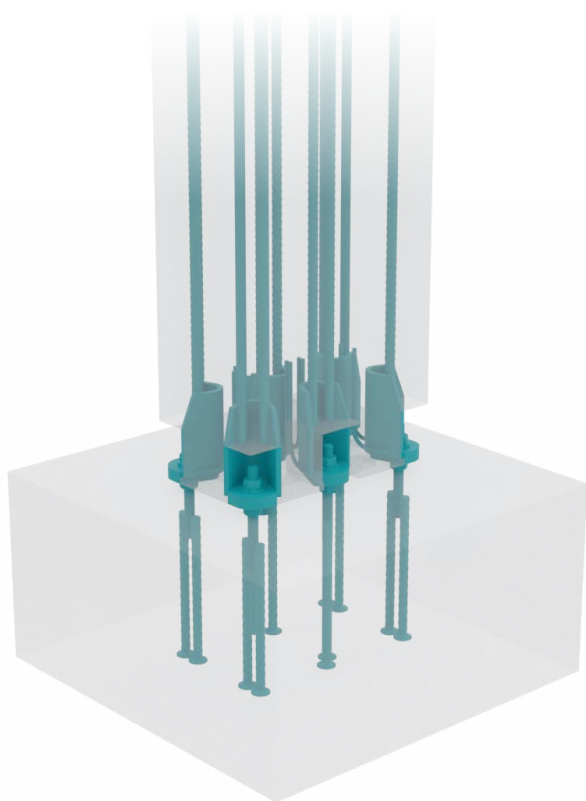
Kuva 1. PPM® L -ankkurointipulttien käyttö betonipilarin liitoksessa anturaan.
