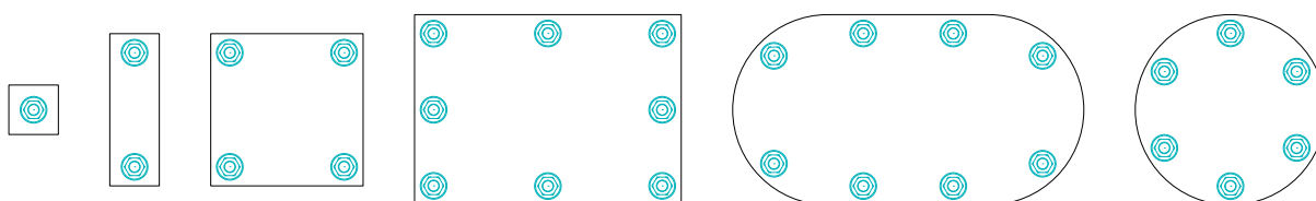
Kuva 5. PPM®-ankkurointipulttien sijoitteluesimerkkejä.
