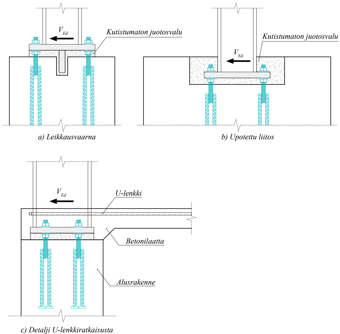
Kuva 15. Yksityiskohtia vaihtoehtoisista leikkausvoiman siirtotavoista.
