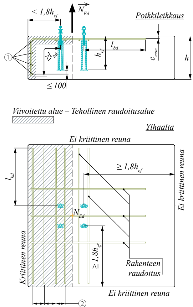
Kuva 10. Halkaisuraudoituksen käyttöesimerkki, kun yksi rakenteen reuna on kriittinen.
