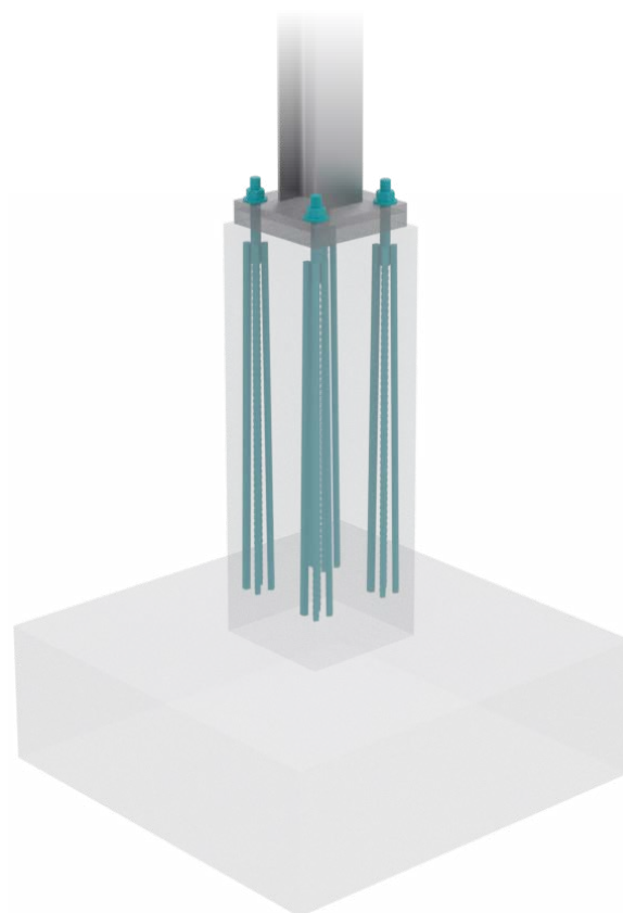
Kuva 2. PPM® P -ankkurointipulttien käyttö teräspilarin liitoksessa peruspilariin.
