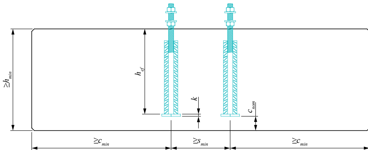
Kuva 6. PPM® L -ankkurointipulttien sijoittaminen perustukseen.
