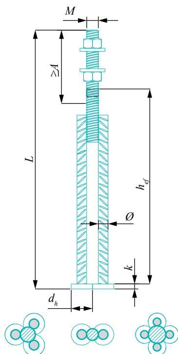
Taulukko 2. PPM® L -ankurointipulttien mitat [mm], painot [kg] ja värimerkinnät.
