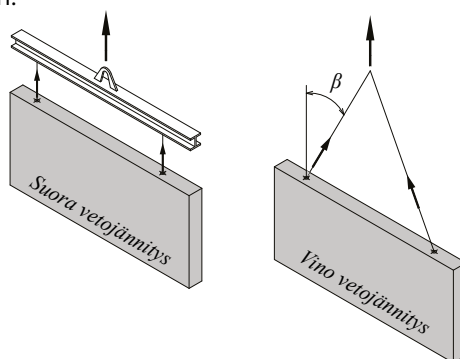
Kuva 18. Sallitut kuormitus suunnat noston aikana.
