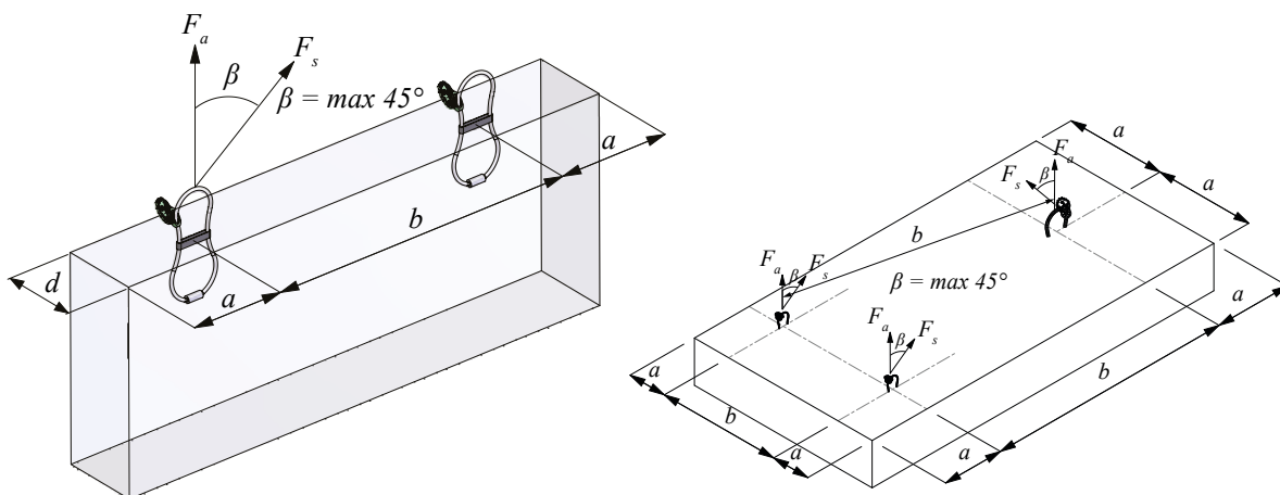
Kuva 8. Kappaleen vähimmäismitat käytettäessä WRA-nostoankkureita.
