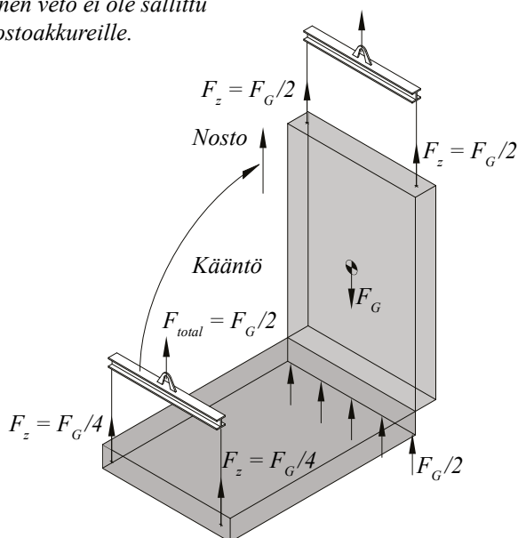
Kuva 20. Nosto vaaka-asennosta pystyasentoon.
