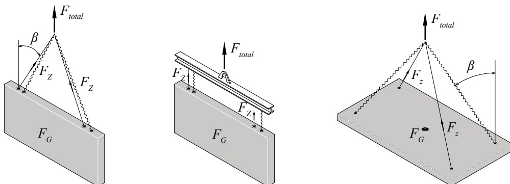
Kuva 14. Tasapainottoman nostotilanne.
