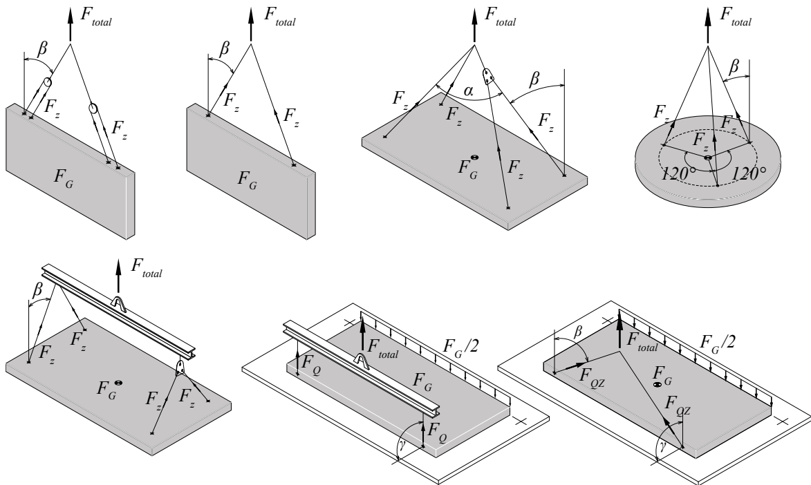
Kuva 13. Tasapainoinen nostotilanne.
