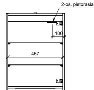
A-A
