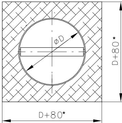
Asennusaukko - neliö
