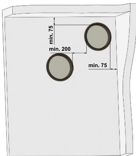
Kuva 2. Rakenteen sisäinen osa (BUILT-IN edge) -mekaanisesti ohjattava tai toimilaitteella varustettu malli
