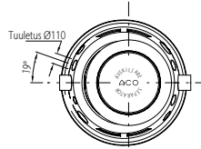
LIPUMAX P-B 8,5/850
