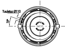
LIPUMAX P-X 4/800
