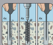
Puhdista reikä puhalla 4x, harjaa 4x, puhalla 4x
