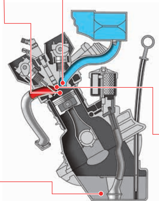
Diesel moottori
