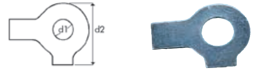
Kaksilehtinen DIN 463
