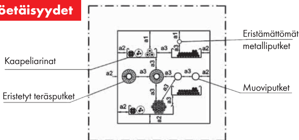
Würth Combo Fire: Reuna- ja keskiöetäisyydet
